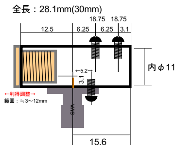
■ディッシュに取り付けた24GHz用ホーン
